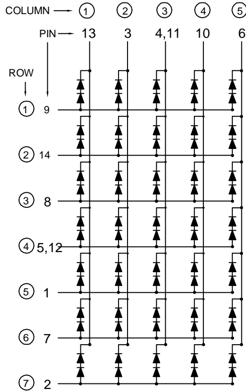
LMD5741BVG-XX
